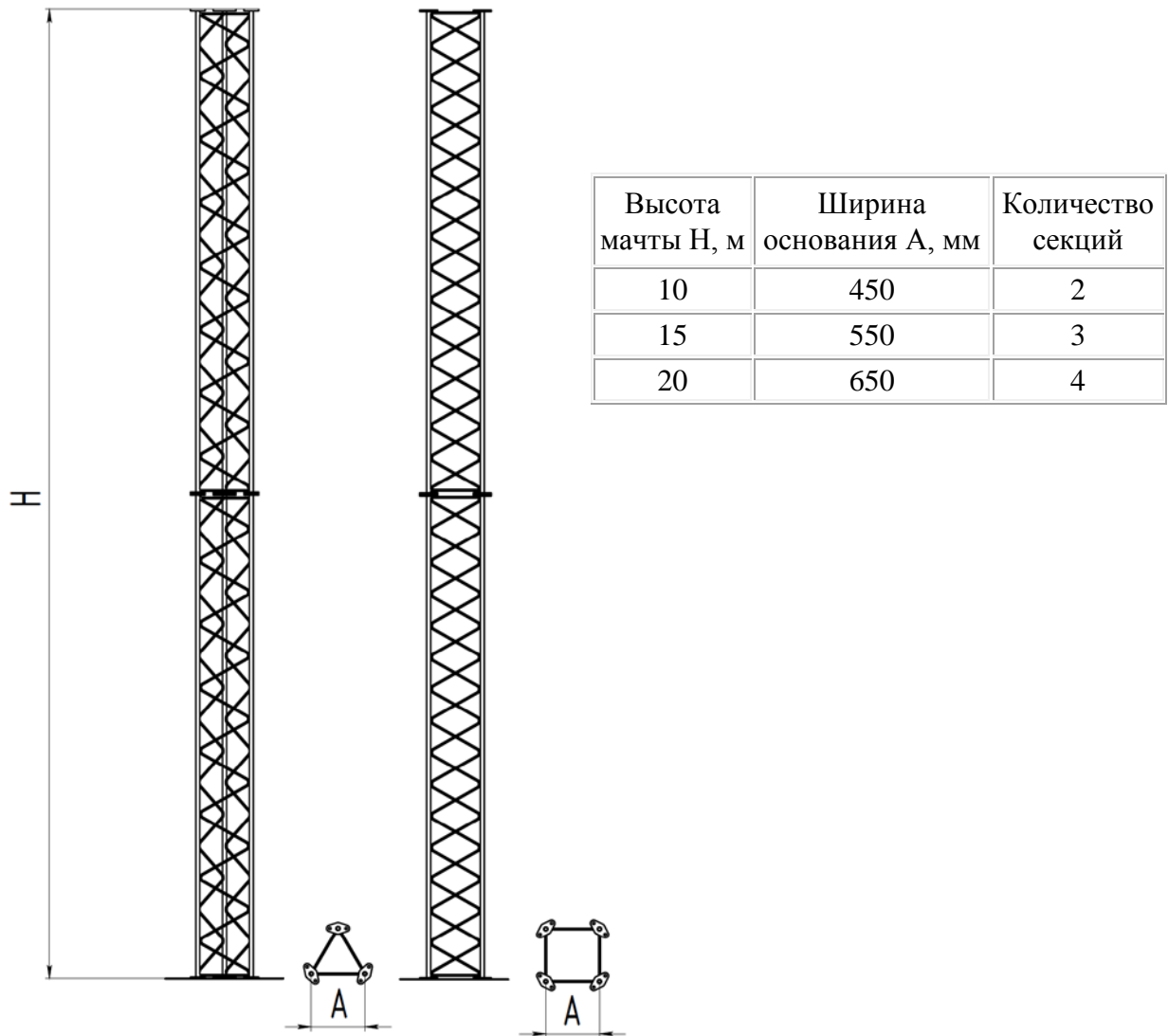
Рис. 1 Стандартные размеры мачты
